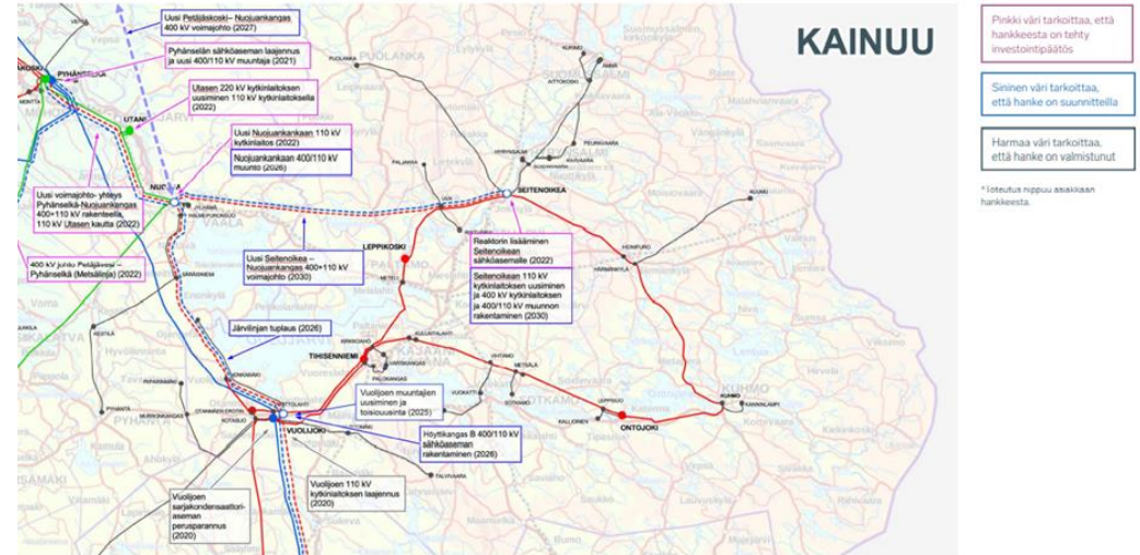
Kuva 28. Fingridin Kainuun alueen kantaverkon kehittämissuunnitelma 2022–2023. Kainuun alueella on runsaasti suunnitella olevia tuulivoimalahankkeita. Laajamittainen tuulivoiman liittäminen vaatii 400 kV verkkoratkaisuja, joiden suunnittelu on käynnissä (kuva: Fingrid 2021)
